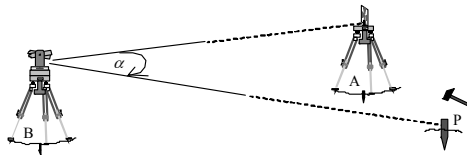
Abb. 11.37a Winkelabsteckung
