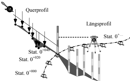
Abb. 11.32b Längs- und Querprofilaufnahme
