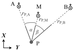
Abb. 11.27b Rückwärtseinschnitt
